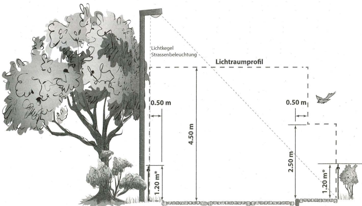
Lichtraumprofil
