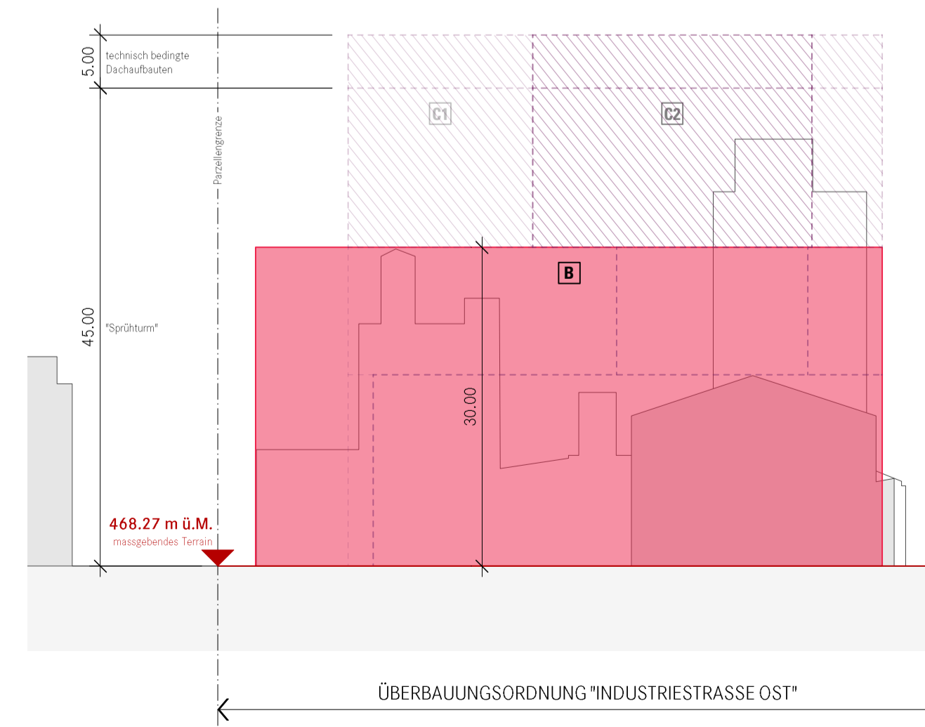
SCHNITT A - A im Mst. 1:500
